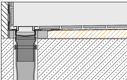
Schlüter®-KERDI-SHOWER-LTS met Schlüter®-KERDI-LINE-V 50 GSE, plaatsing tegen wand
