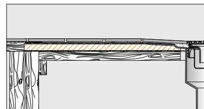
Inbouwvoorbeeld Schlüter®-KERDI-SHOWER-TT
