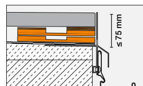
Randprofiel Schlüter®-BARA-RKLT
