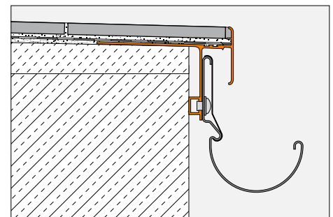
Opbouw met Schlüter-DITRA en Schlüter-BARA-RTKEG
